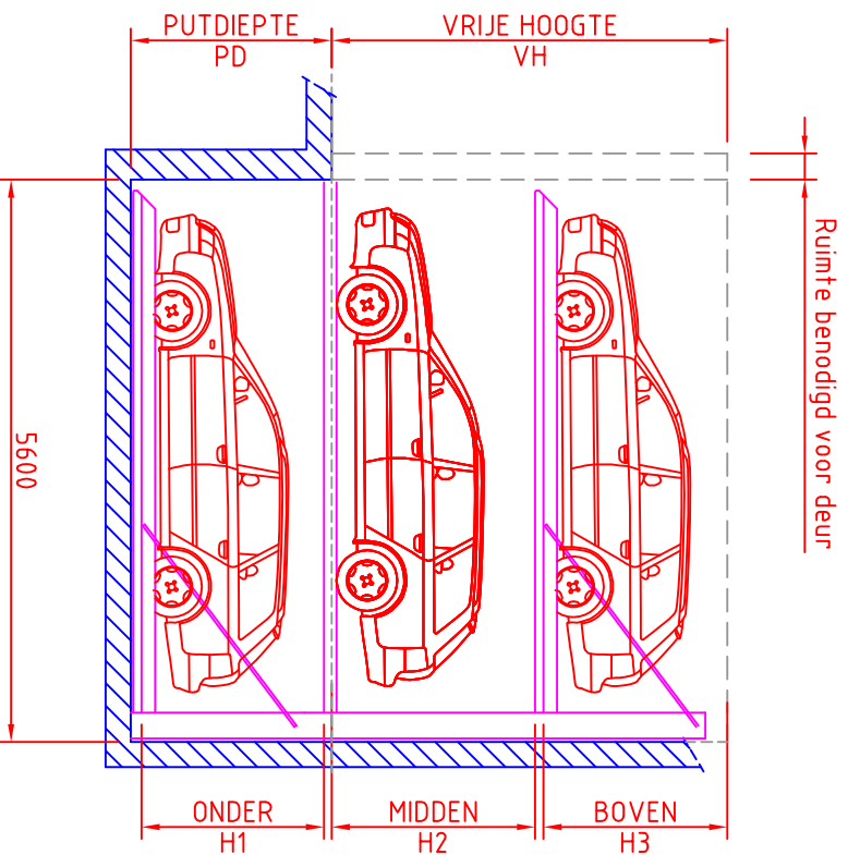
Langsdoorsnede
