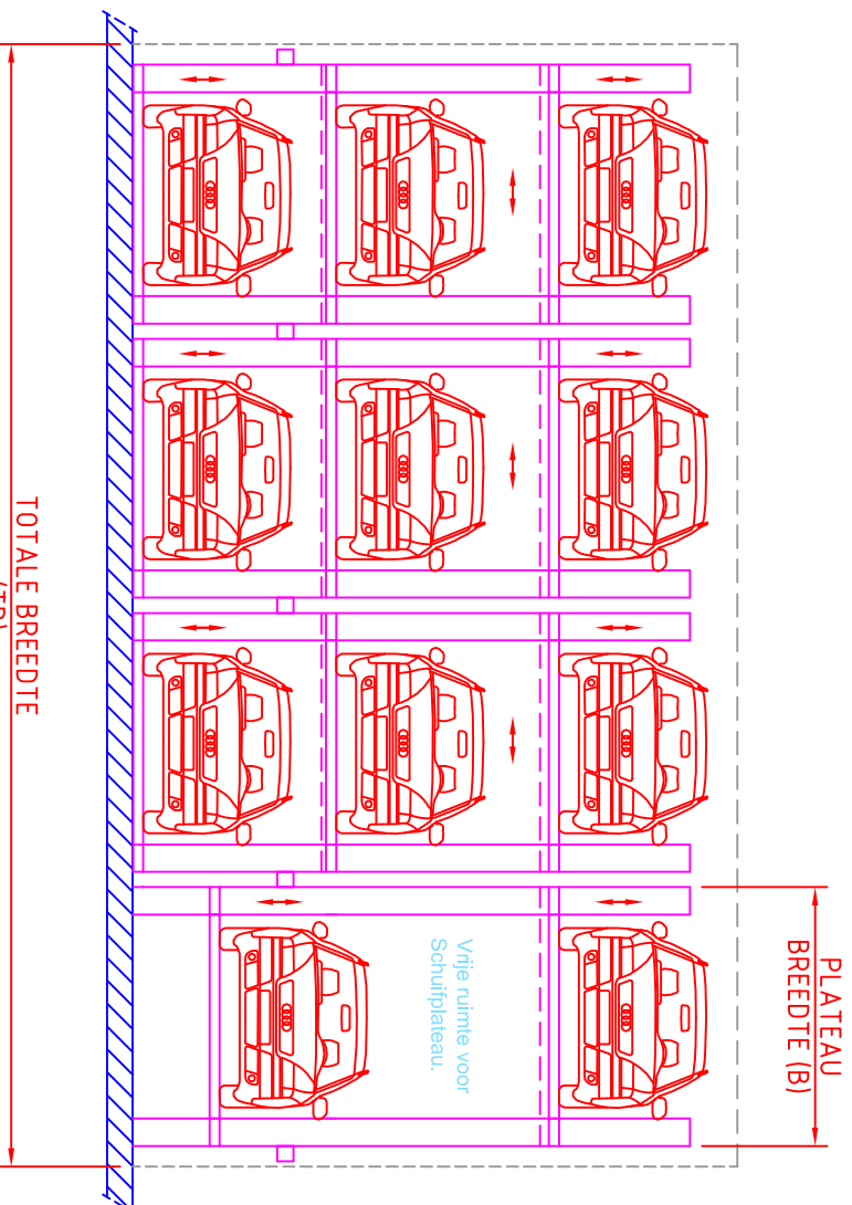
Dwarsdoorsnede
