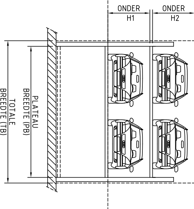
Dwarsdoorsnede CP2404
