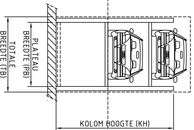
Dwarsdoorsnede CP2402
